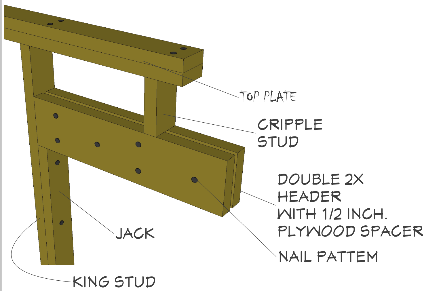
DOOR HEADER DETAIL S-4
